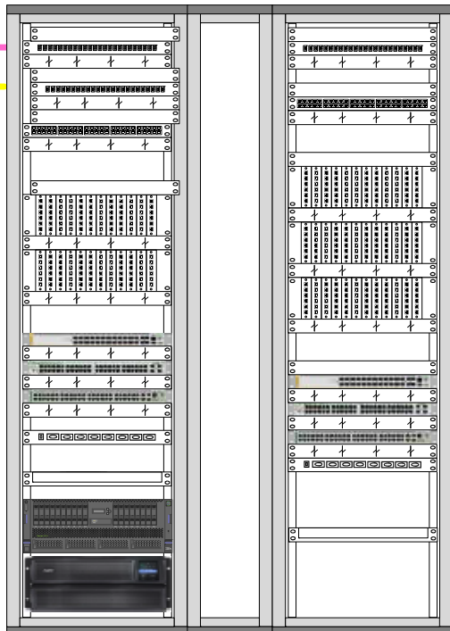
Gebäudeverteiler
