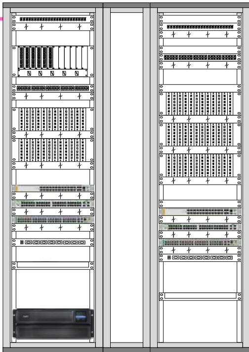
Etagenverteiler
