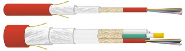
Figure 4 : Des câbles FO Universal Safety de Datwyler sont testés pour le maintien de fonction pour un maximum de 30 minutes selon la norme DIN 4102-12.
